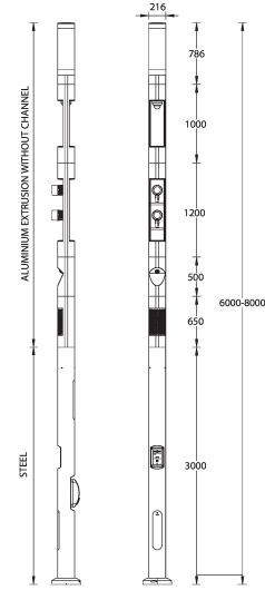
LCP-S0216
