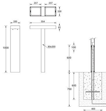
LI-10032-SB
